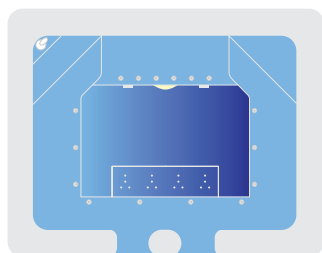
LAP SPA D. ext./ 2,90 x 2,25 x 0,95 m. P. máx./ 1,10 m. Ancho bordillo/ 0,25 m.
