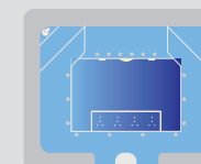
LAP SPA D. ext./ 2,90 x 2,25 x 0,95 m. P. máx./ 1,10 m. Ancho bordillo/ 0,25 m.
